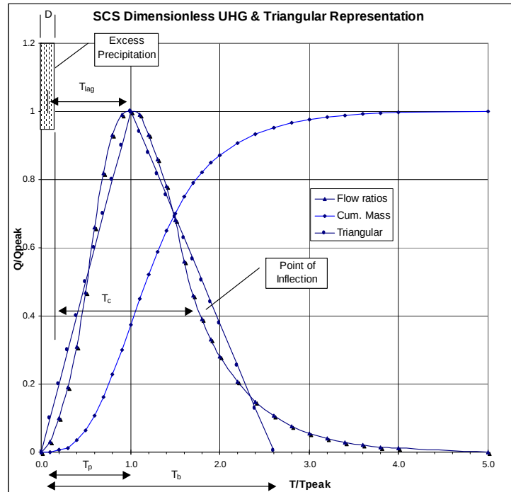
Figura 2: IUH-SCS
